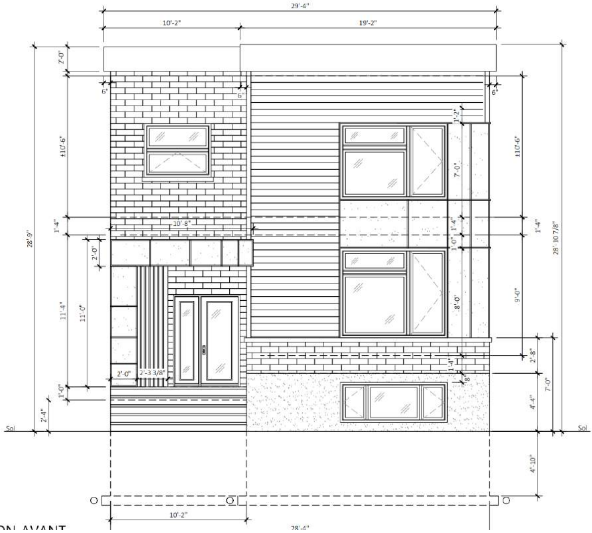
ÉLEVATION AVANT
